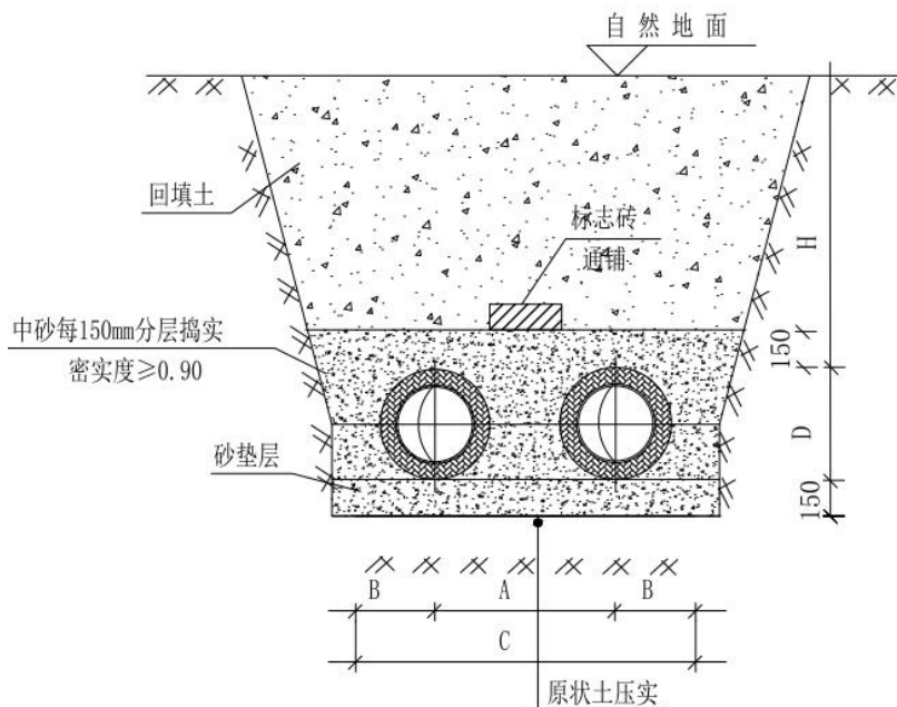
图 8 供热管道横断面图
