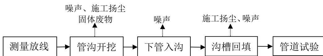
图 7 天然气管道施工工艺流程及产污环节图
