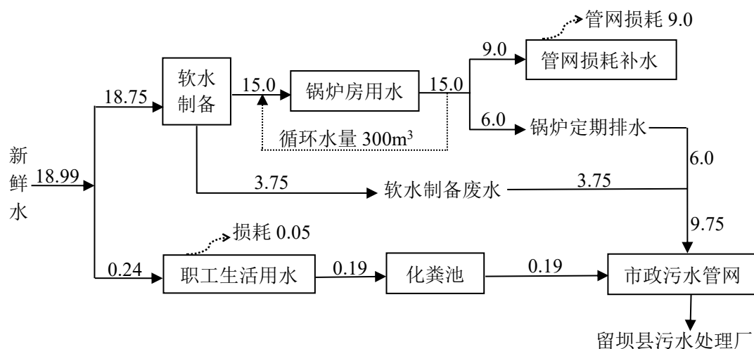
图4 本项目水平衡图 单位: \text{m}^3/\text{d}
