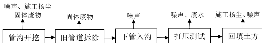
图 6 供热管线施工工艺流程及产污环节图
