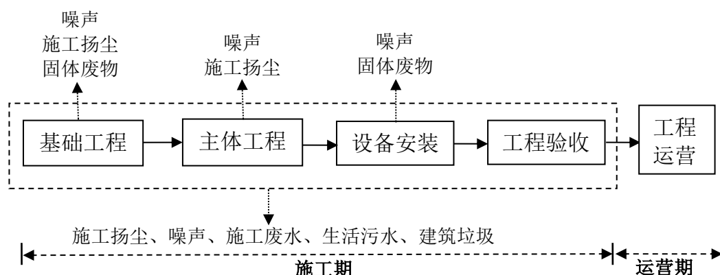
图 5 供热站施工工艺流程及产污环节图
