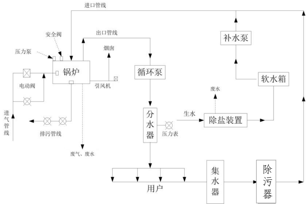
图 9 本项目供热站生产工艺流程及产污环节图
